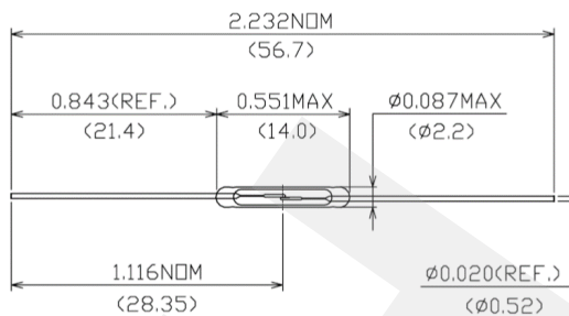
■外形寸法图(单位: mm) 外形尺寸图(单位: mm)
