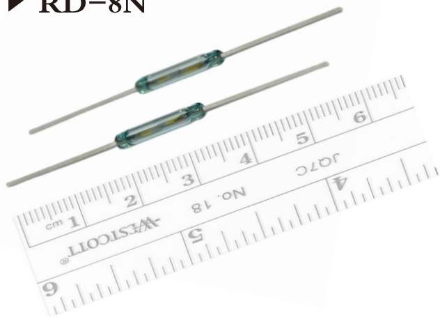
■外形尺寸图(单位: mm) 外形尺寸图(单位: mm)
