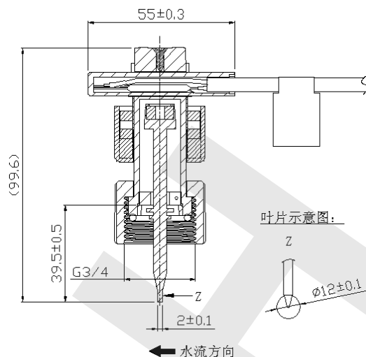
■外形尺寸图(单位: mm) 外形尺寸图(单位: mm)
