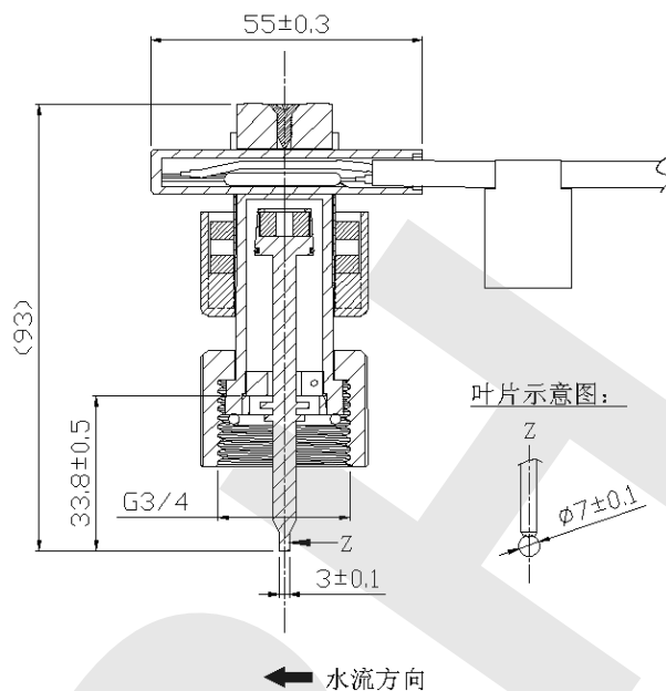
■外形尺寸图(单位: mm) 外形尺寸图(单位: mm)
