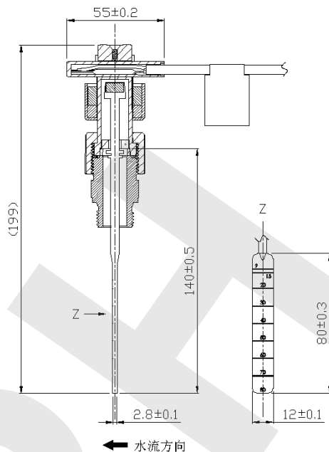
■外形尺寸图(单位: mm) 外形尺寸图(单位: mm)
