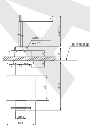
■外形寸法図(単位: mm) 外形尺寸图(单位: mm)
