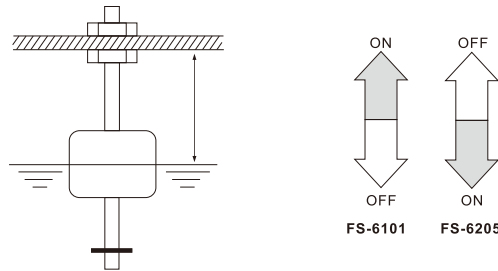
■動作特性/OPERATING CHARACTERISTICS 动作特性
